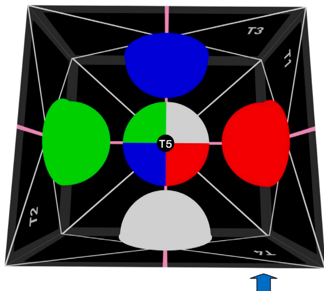
Figura 2 – Simulação de visão superior e disposição das telas na sala
