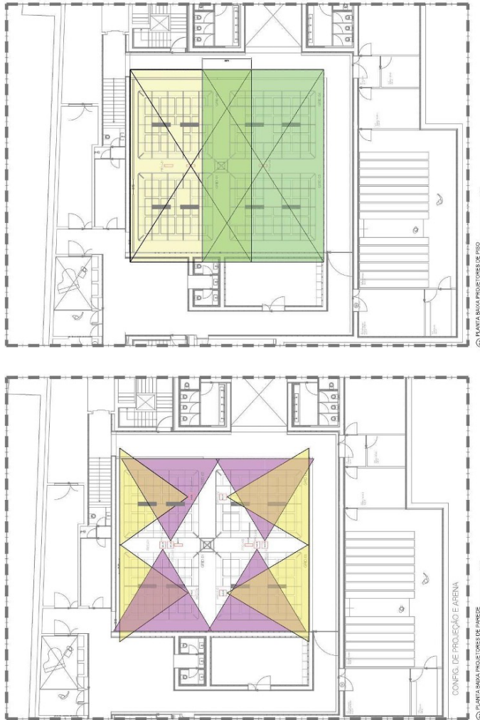
Figura 4 – Planta baixa da Sala Imersiva
