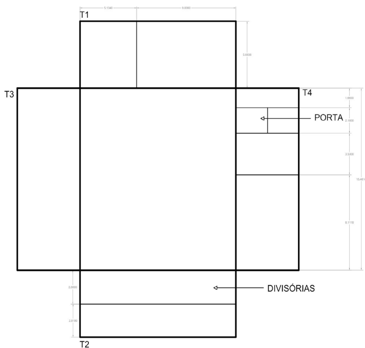
Figura 3 – Área das telas
